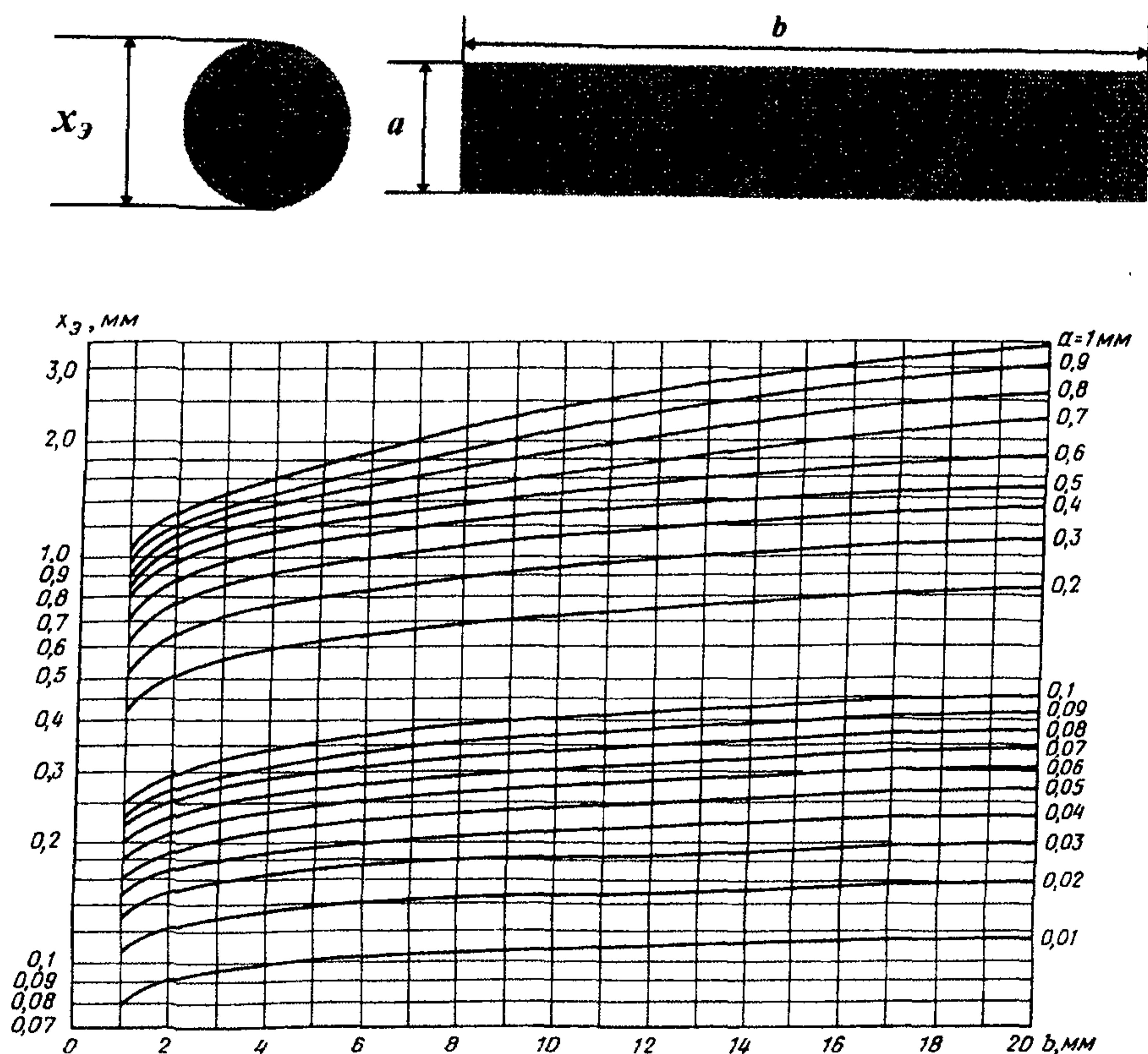
Рисунок Г.1 — Номограмма для определения эквивалентного размера протяженных объектов различия при расстояниях от глаза до объекта до 500 мм
